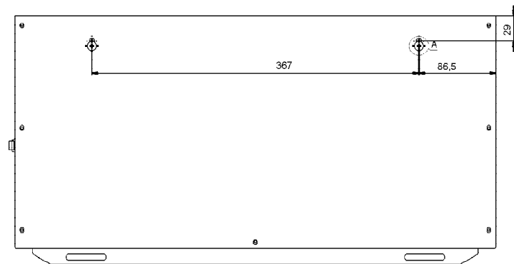
Габаритные и установочные размеры стабилизатора напряжения переменного тока LIDER PS5000SQ-15
