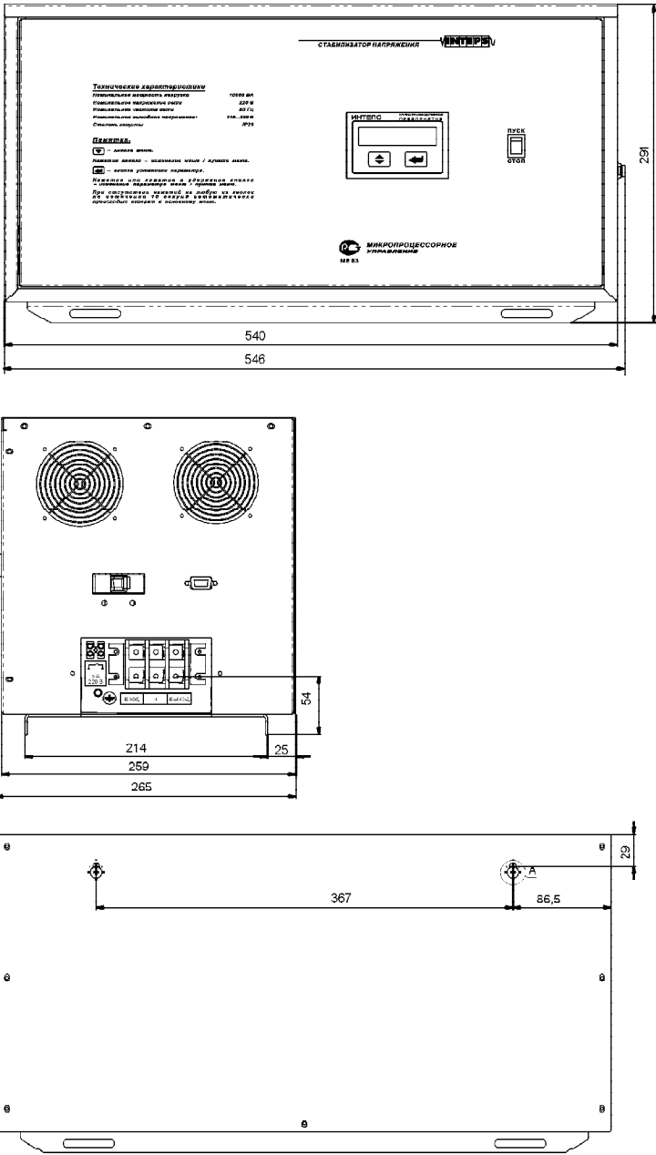
Габаритные и установочные размеры стабилизатора напряжения переменного тока LIDER PS5000SQ-40
