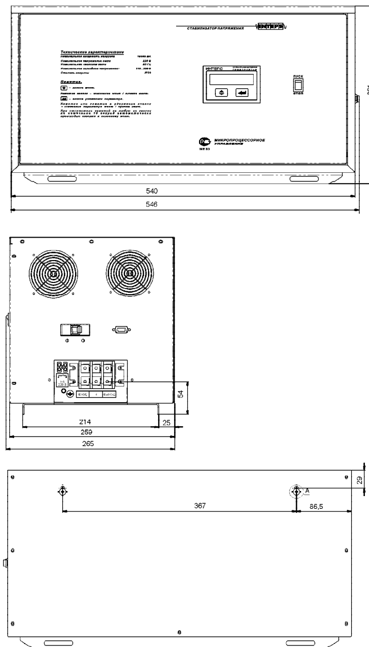
Габаритные и установочные размеры стабилизатора напряжения переменного тока LIDER PS5000SQ-15
