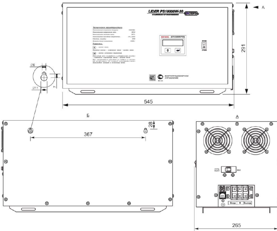
Габаритные и установочные размеры стабилизаторов напряжения переменного тока LIDER PS3000W-50
